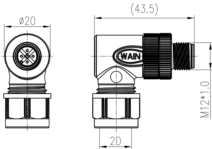
电缆直径:2D5 Cable outlet:2D5
